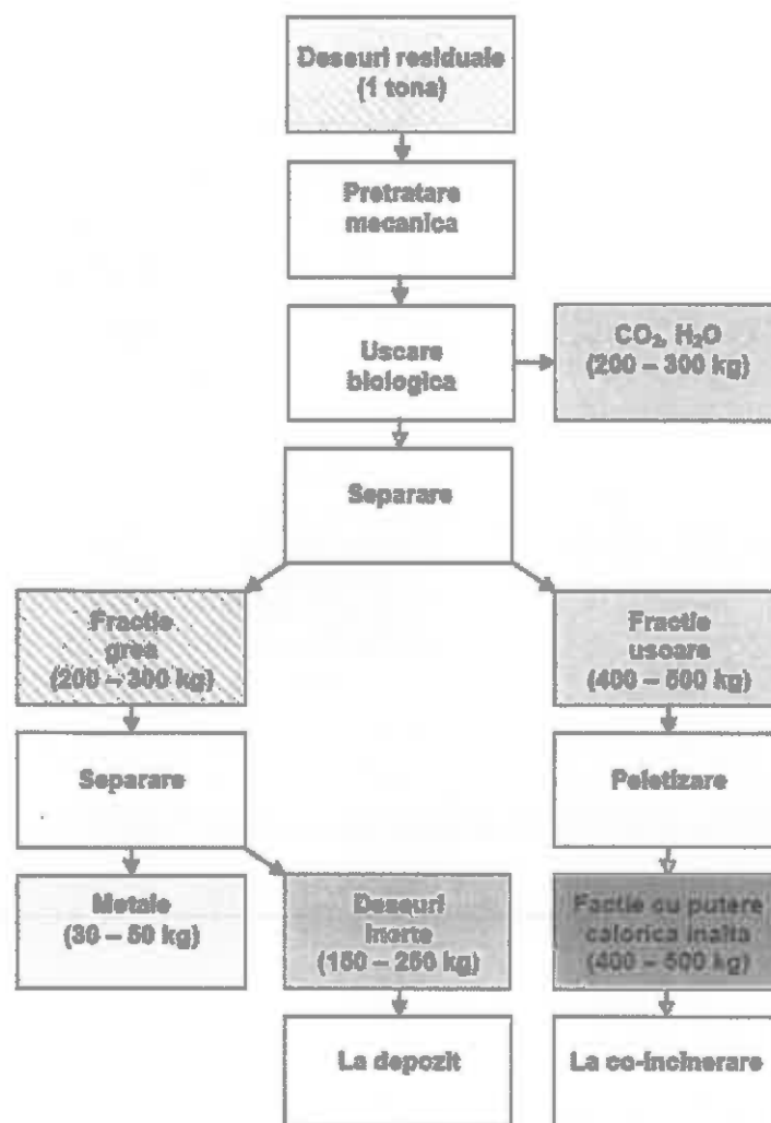
Figura nr. 2 - Schema instalației de tratare mecano-biologică cu bio-uscare și producere de RDF
